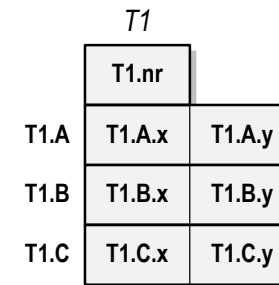
Rys. 5. Zmienna strukturalna T1 zawierająca cztery pola
