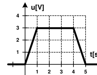
Rys. 1. Przebieg impulsu trapezowego
