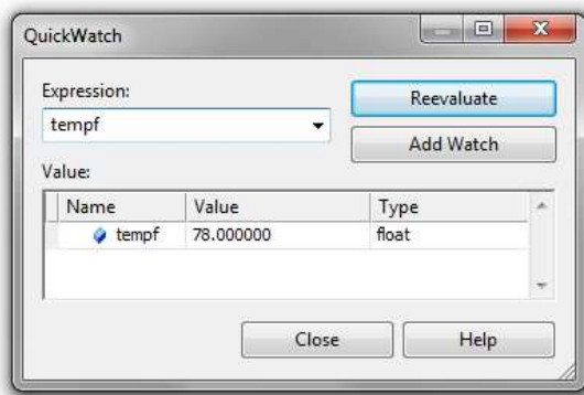
Rys. 8. Okno QuickWatch
