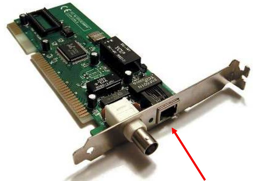
Karta sieciowa ze złączem 8P8C
