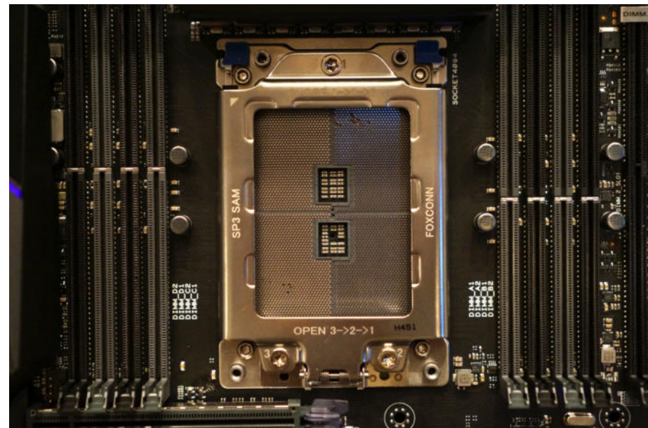
Socket TR4
