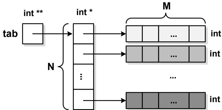
Rys. 7. Implementacja macierzy w postaci wskaźnika do tablicy wskaźników
