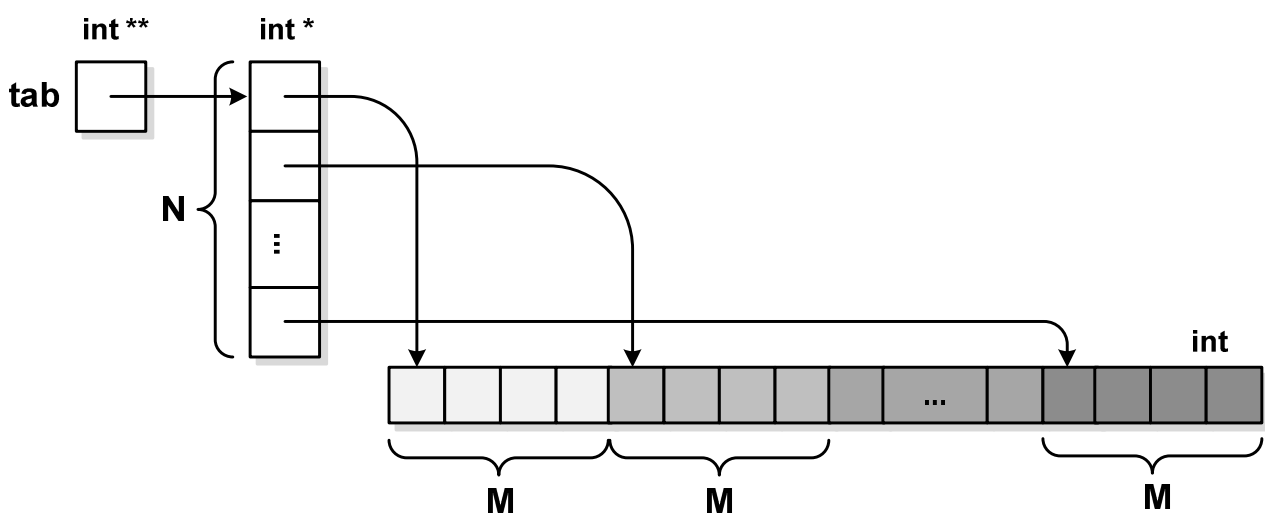
Rys. 8. Implementacja macierzy w postaci wektora N \times M - elementowego i wektora wskaźników
