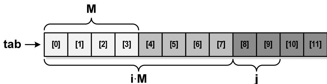
Rys. 6. Macierz w postaci wektora N×M - elementowego
