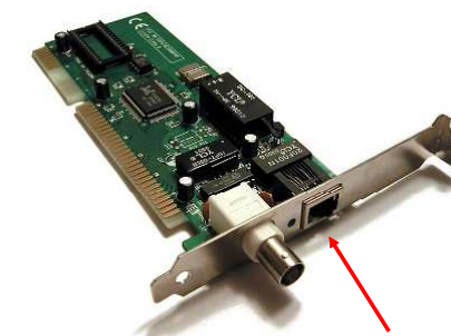
Karta sieciowa ze złączem 8P8C
