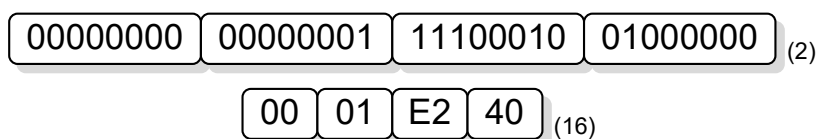
Rys. 1. Sposób przechowywania liczby całkowitej 123456 (typ int) w pamięci komputera (zapis w systemie dwójkowym i szesnastkowym)
