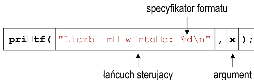
Rys. 1. Struktura funkcji printf()
