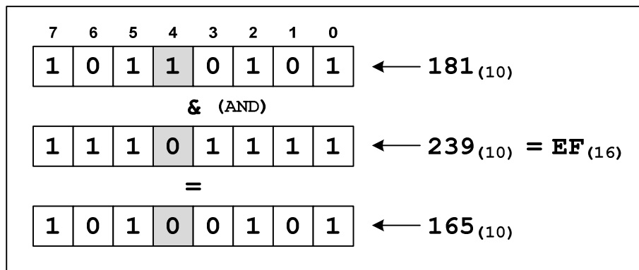
Rys. 3. Wyzerowanie wybranego bitu w bajcie
