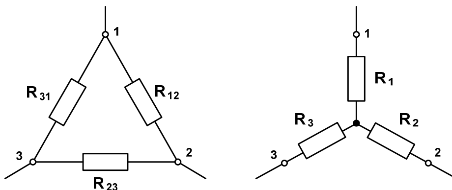
Rys. 3 Trójkąt i gwiazda rezystancji
