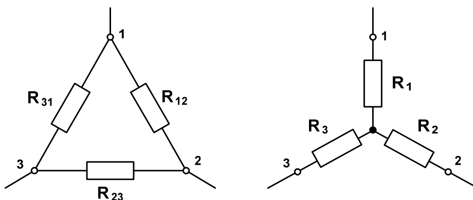
Rys. 3 Trójkąt i gwiazda rezystancji
